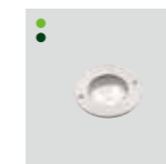
HBD-D095 W142xD142xH203mm 3.1W 3000K 263lm
